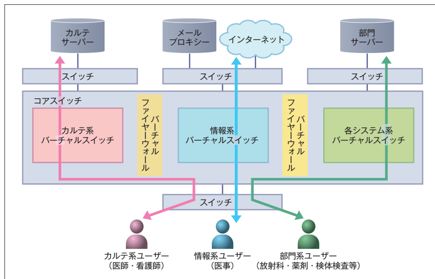
院内仮想ネットワーク図
